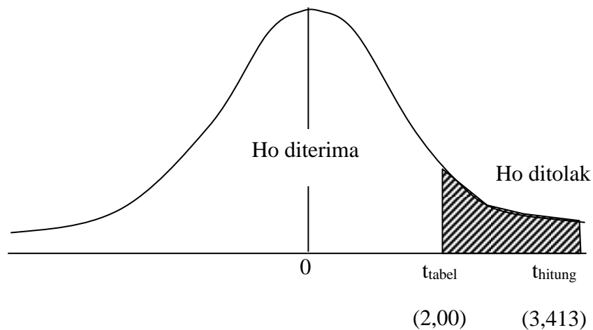
Gambar 3. Kurva Distribusi Normal t-testkedua (Sumber: Lampiran 6, 2022)
