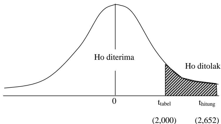
Gambar 2. Kurva Distribusi Normal t-test pertama
