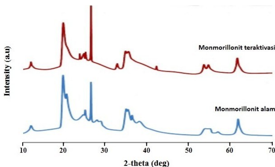
Gambar 2. Pola XRD monmorillonit alam dan teraktivasi
