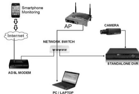
Gambar 1. Topologi Jaringan CCTV [3]
