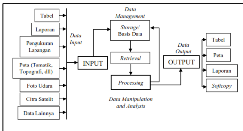
Gambar 1. Subsistem dalam SIG
