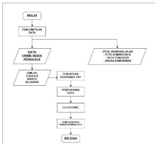
Gambar 3. Perancangan Pemetaan menggunakan SIG
